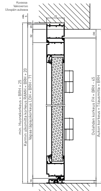
Pystyleikkaus (asennus aukon taakse)
