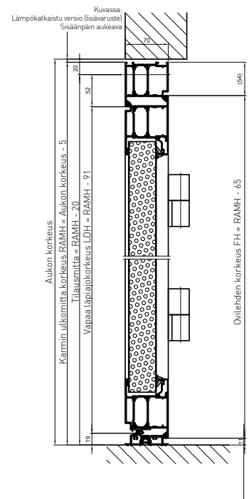
Pystyleikkaus (asennus aukkoon)
