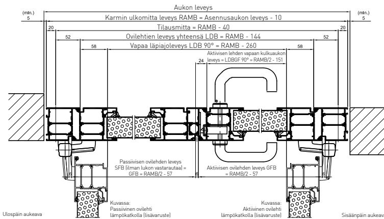
Vaakaleikkaus (asennus aukkoon)
