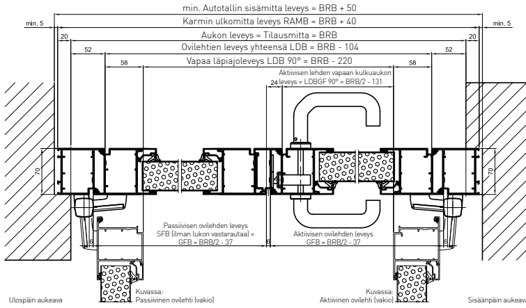
Vaakaleikkaus (asennus aukon taakse)
