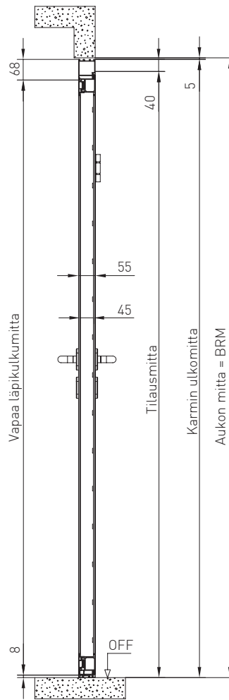
Pystyleikkaus/Asennus aukkoon
